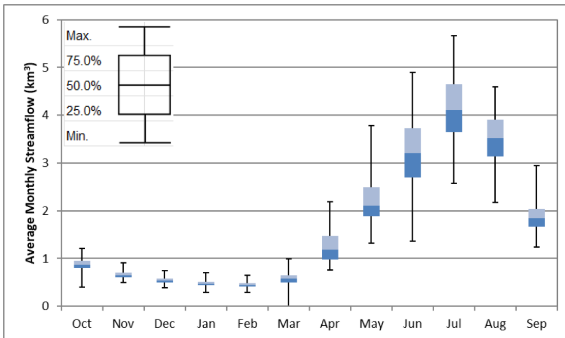
Расми 13-5: Диаграммаи Box and Whisker барои ҷараёни моҳонаи об дар НБО Роғун
