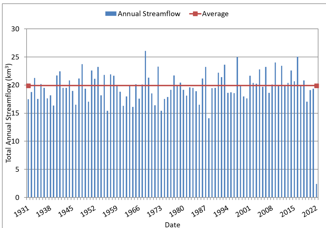
Расми 13-6: Ҷараёни солонаи дарёи Вахш дар НБО Роғун
