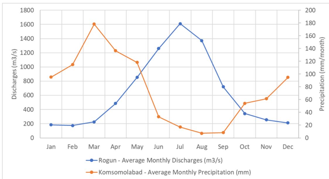
Расми 13-4: Боришоти миёнаи моҳона ва ҷараёни миёнаи дарёи Вахш
