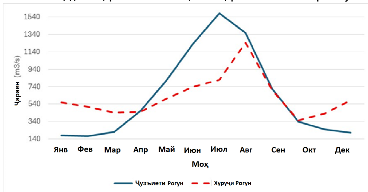
Расми 3-16 - Ҷадвали ҷараени миёнаи моҳона ва ҷараени об аз обанбори Роғун
