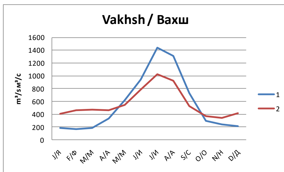
Расми 13-8: Аъсири сарбанди Норақ ба ҷараёни дарёи Вахш
