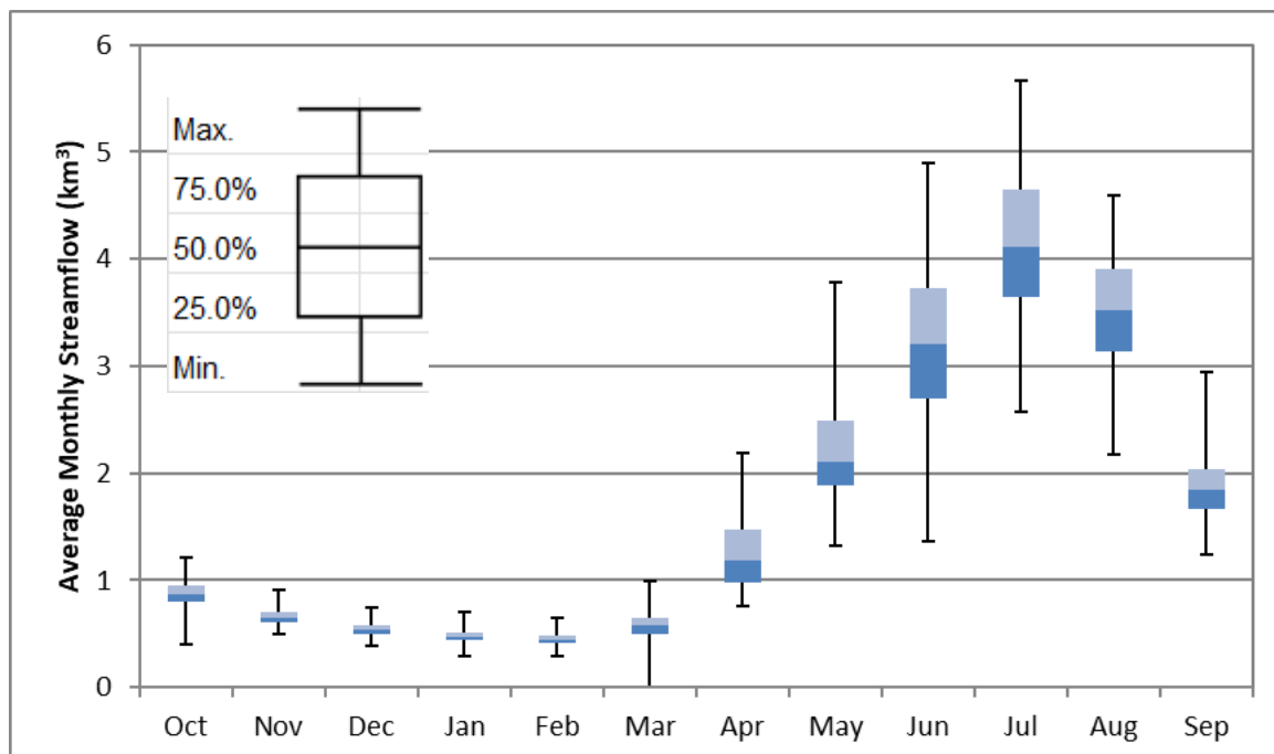
Расми 3-15 - Графики росткунҷаи обгузарони моҳонаи нерӯгоҳи барқи оби Роғун
