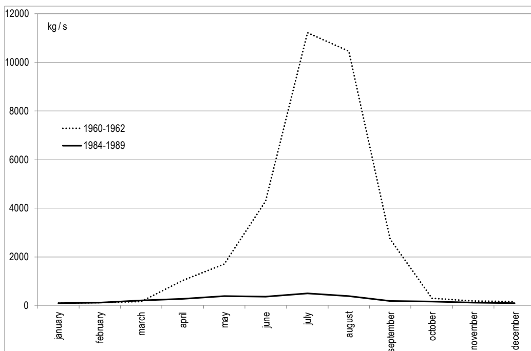
Расми 13-20: Зарраҳои муаллақ — Бешаи палангон, Вахш, пеш ва баъд аз ба кор даромадани НБО Норак
