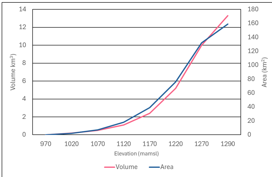
Расми 13-11: Графики масоҳат-ҳаҷми обанбори Роғун
