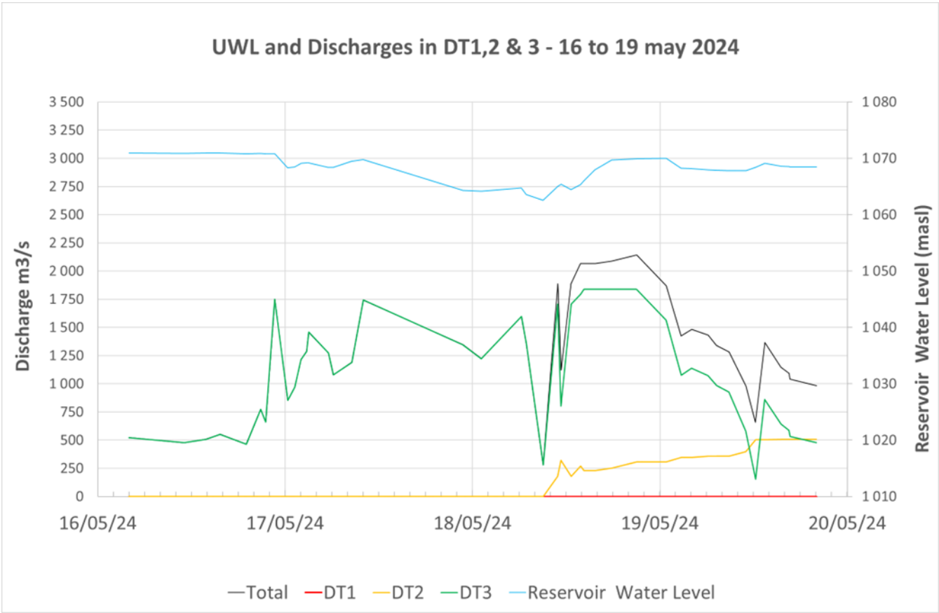
Расми 13-23: Сатҳи обанбор ва холишавии обхезӣ тавассути нақбҳои поёнӣ.
