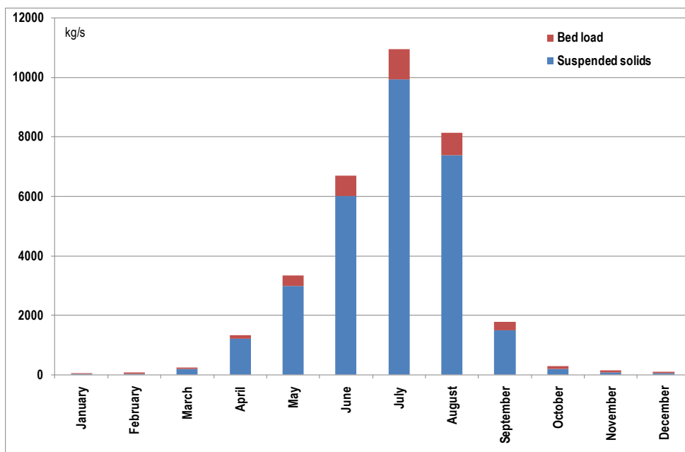
Расми 13-19: Зарраҳои муаллақ ва таҳшинҳо дар қаър дар дарёи Вахш дар Роғун (2010)
