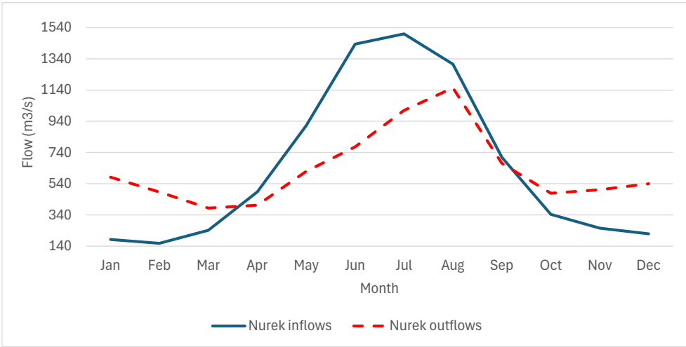
Расми 13-9: Ҷараёнҳои воридшаванда ва хориҷшавандаи миёнаи моҳона дар НБО Норак дар ҳолати истифодабарии ҷорӣ
