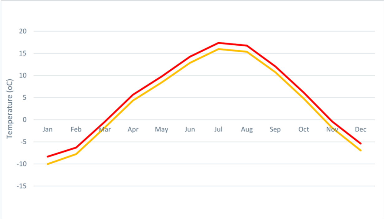
Расми 9-6 – Ҳароратҳои миёнаи моҳона
