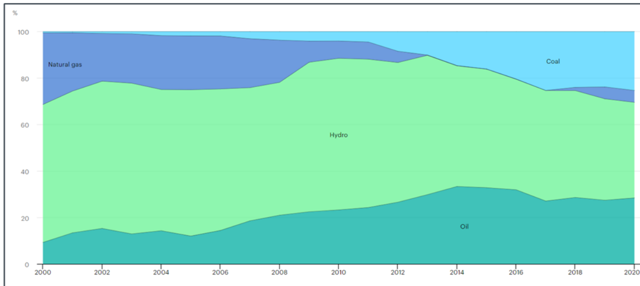
Расми 4-1 - Ҳаҷми умумии таъминоти барқ дар тақсимои манбаъҳо, Тоҷикистон, солҳои 2000-2020
