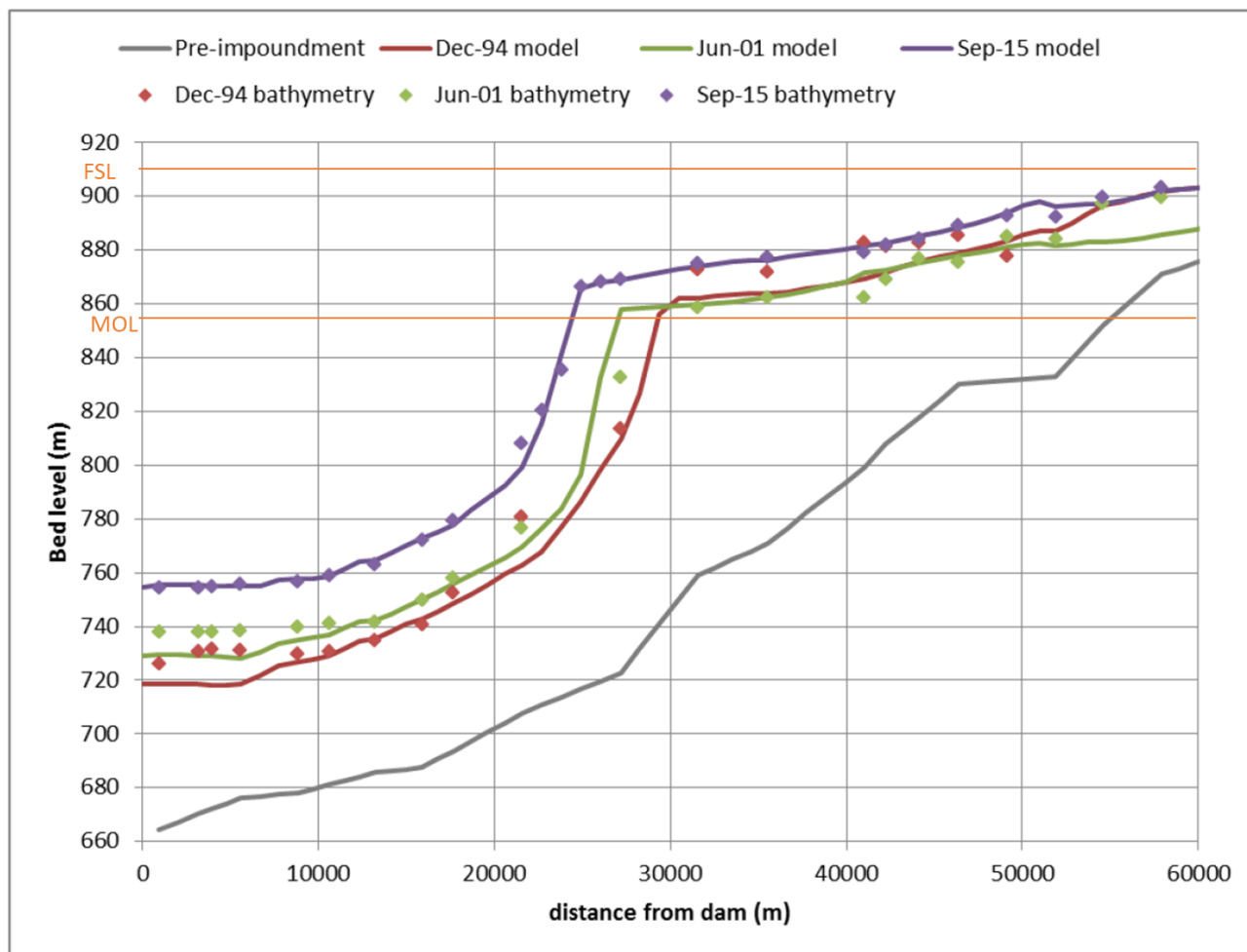
Расми 13-21: Таҳшиншавӣ дар обанбори Норақ
